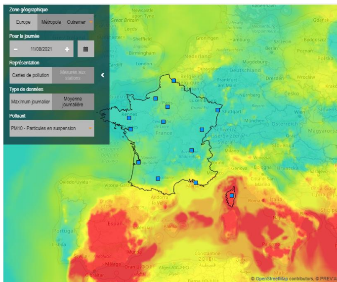
Carte de prévision PREV'AIR pour le 11/08/2021
